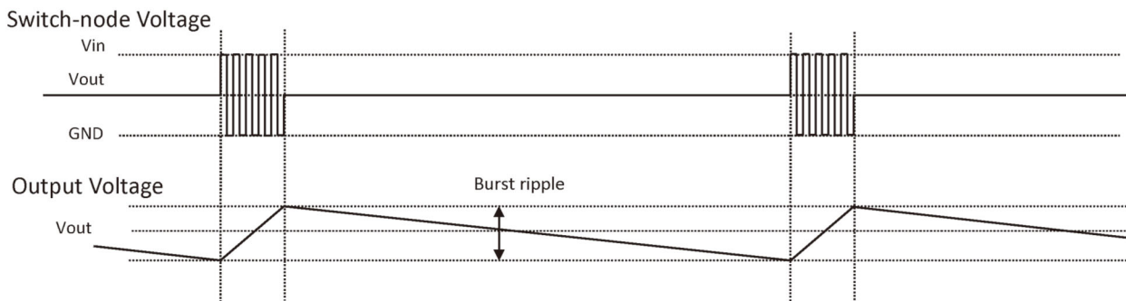
图 2 LTC3890 突发模式工作的电压时序图
