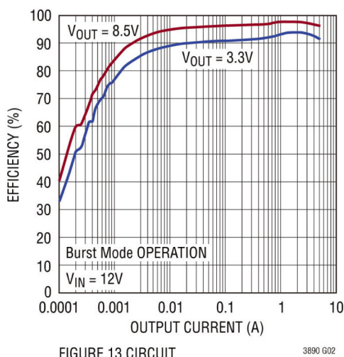
图 3 从 12V 输入至 8.5V 和 3.3V 输出时 LTC3890 的效率曲线
