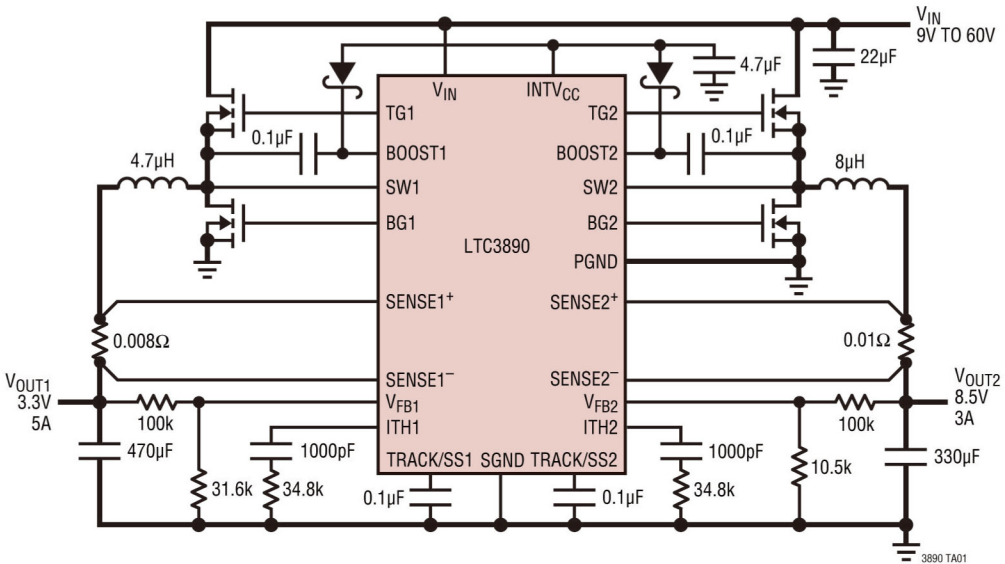
图 1 将 9V 至 60V 输入转换为 8.5V/3A 和 3.3V/5A 输出的 LTC3890 原理图
